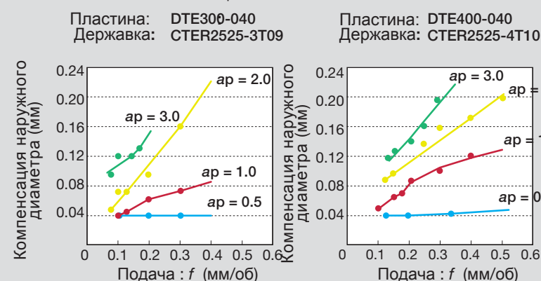
Рис. 2 Величина компенсации
